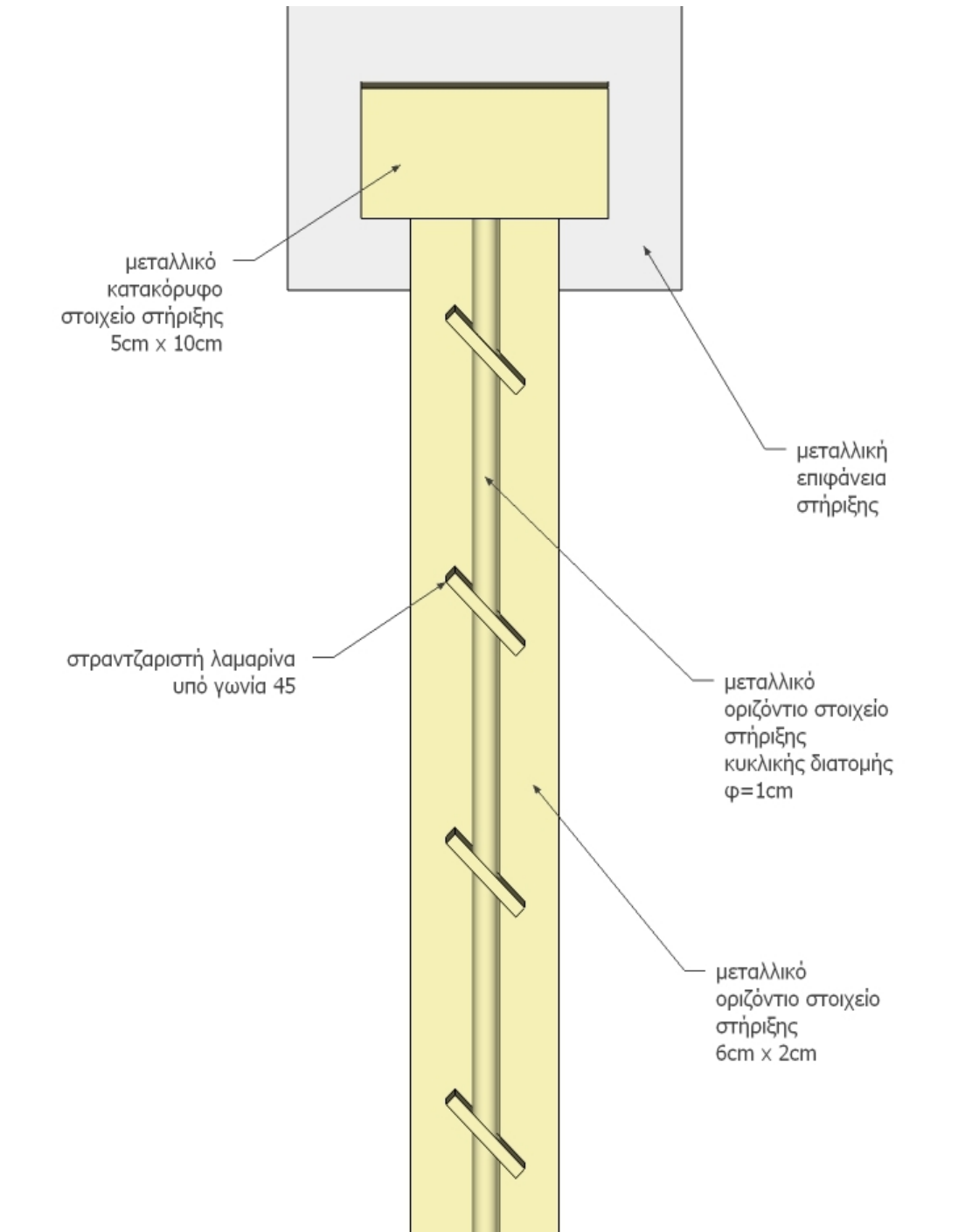
ΕΙΚΟΝΑ 4. ΛΕΠΤΟΜΕΡΕΙΑ PANEL. ΚΑΤΟΨΗ.
